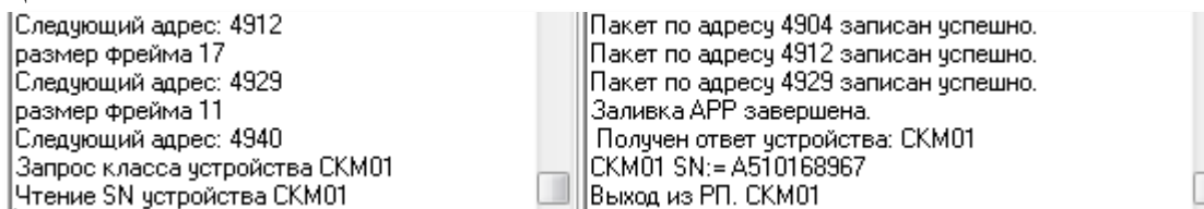
Рис.19.14 Завершение заливки АПП в СУ СКМ01.
