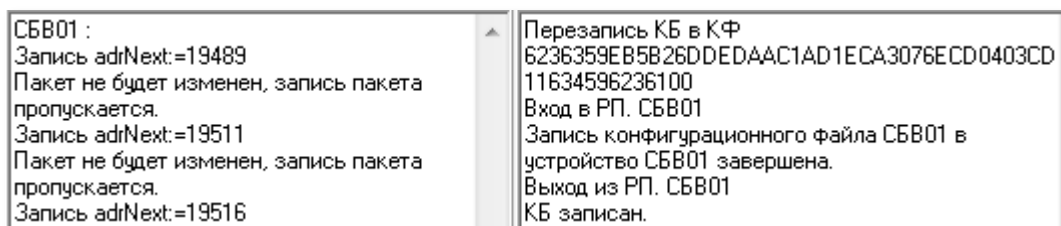
Рис.19.19 Пример записи КБ в СБВ02.
