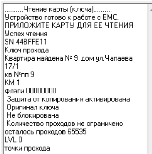
Рис.18.18 Результат чтения ключа прохода.
