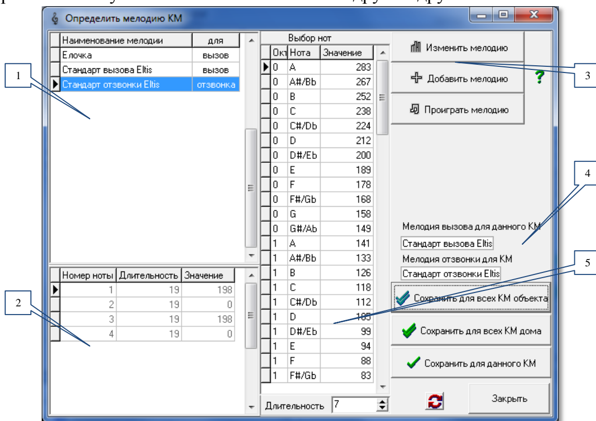
Рис.10.7 Окно «Определить мелодию KM» (пример).
