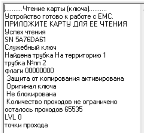
Рис.18.19 Чтение служебного ключа.
