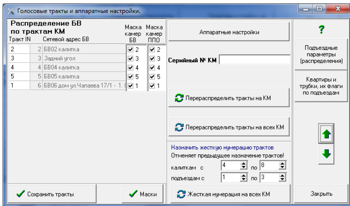
Рис.10.3 Окно «Голосовые тракты и аппаратные настройки».
