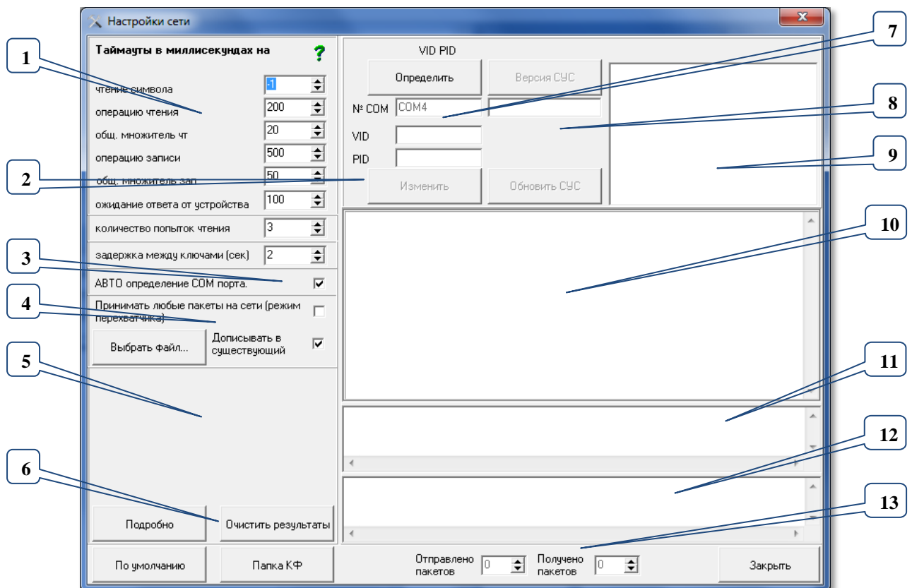
Рис.16.2 Окно настроек сети при отключенной сети.
