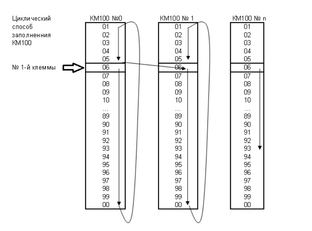
Рис 10.12 Пример циклического заполнения клемм KM100 при номере первой квартиры «6».
