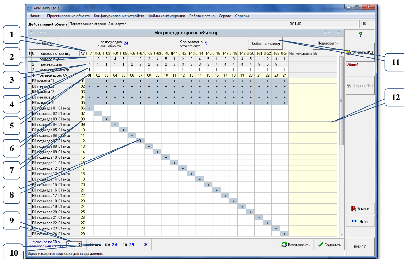
Рис.8.7 Первичное окно незаполненной матрицы (пример).
