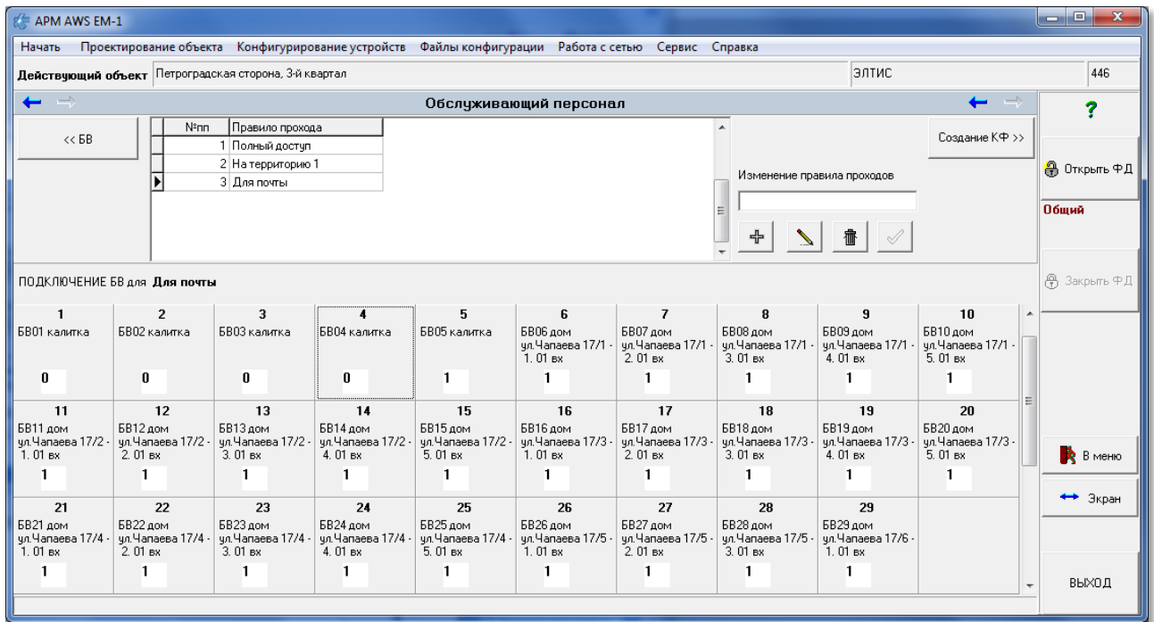
Рис.12.4 Пример окна правил прохода после корректировки маски БВ.
